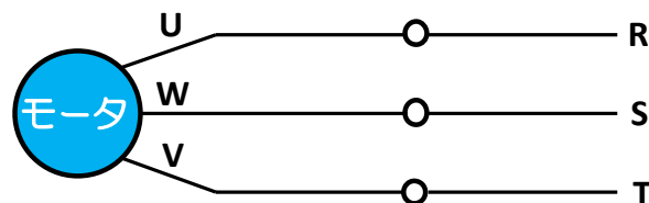
【図A】（逆相結線）
