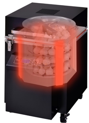
側面 4 方向に搭載された加熱ヒーター(イメージ)
